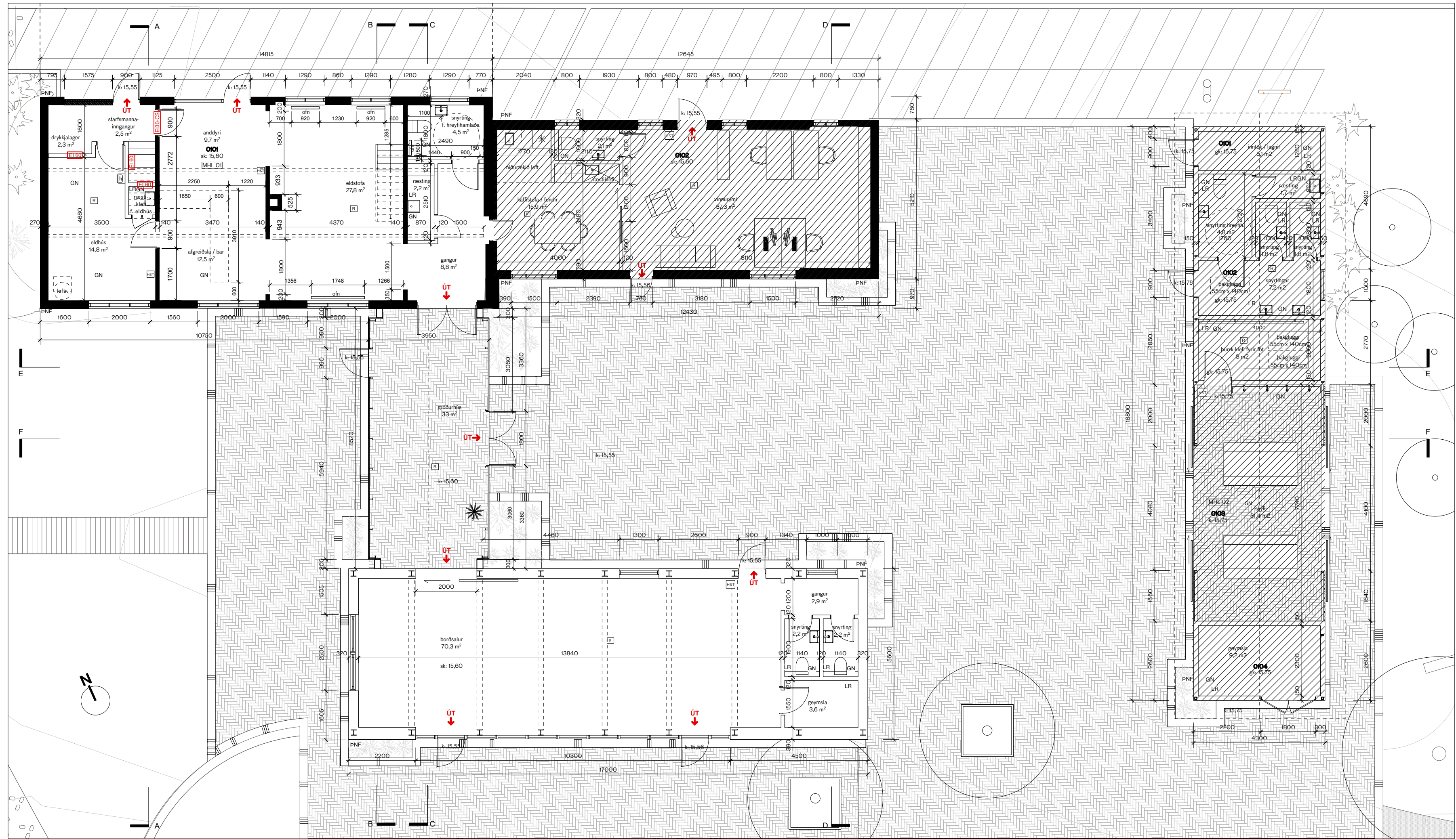
GRUNNMYND 1.HÆÐAR 1:100
