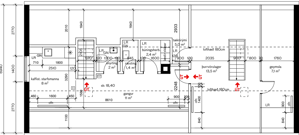
GRUNNMYND RISHÆÐAR 1:100
